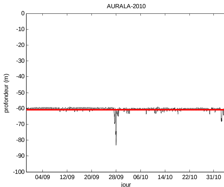
Figure 4 : profondeur de l'hydrophone AURAL A au cours de la période d'enregistrement
