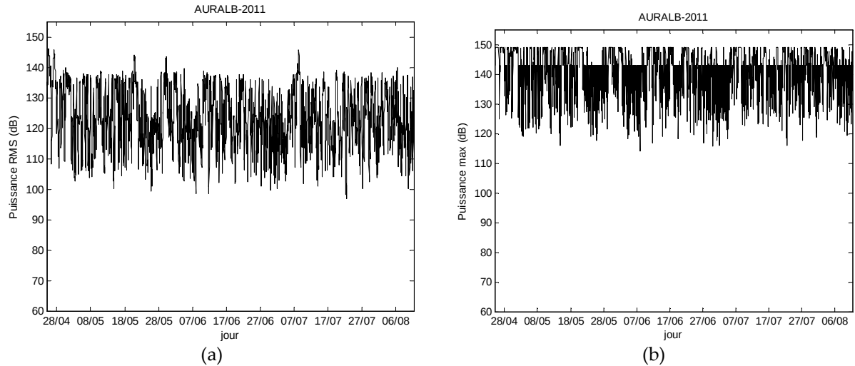
Figure 26 : évolution de la puissance au cours des enregistrements a) puissance RMS et b) puissance max
