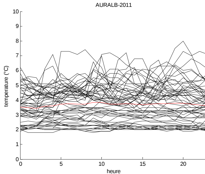
Figure 15 : évolution de la température en fonction de l'heure du jour
