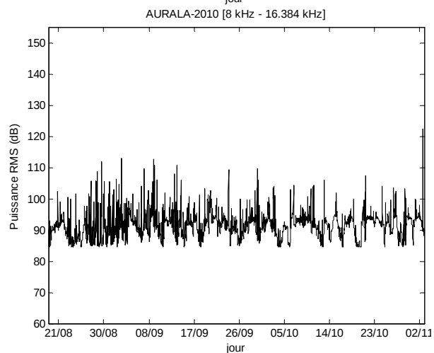
(a) (b) Figure 21 : évolution de la puissance au cours des enregistrements dans les différentes bandes fréquentielles a) puissance RMS et b) puissance max
