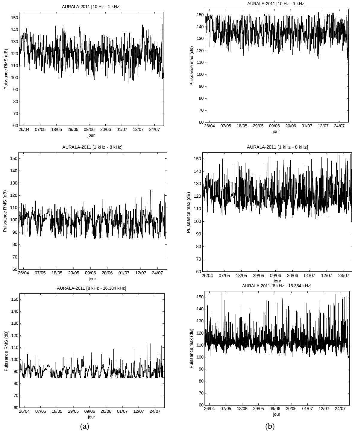
Figure 25 : évolution de la puissance au cours des enregistrements dans les différentes bandes fréquentielles a) puissance RMS et puissance max
