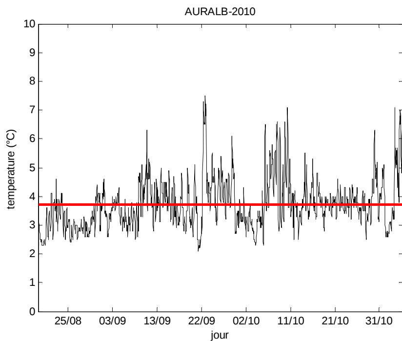
Figure 8 : variation de température pendant la période d'enregistrement
