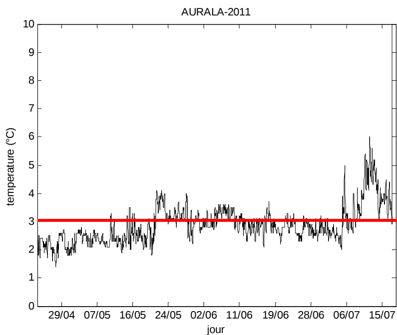
Figure 11 : température pendant la période d'enregistrement
