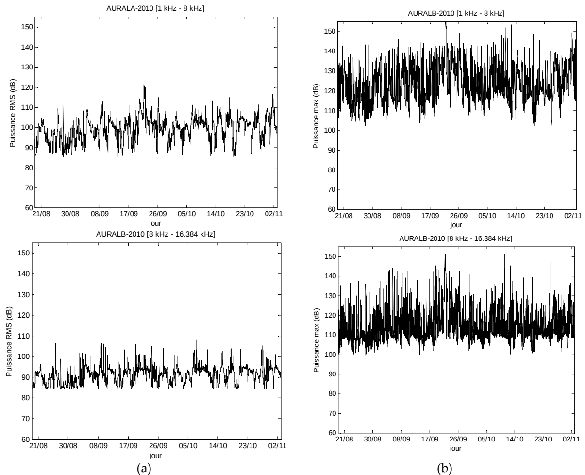
(a) (b) Figure 23 : évolution de la puissance au cours des enregistrements dans les différentes bandes fréquentielles a) puissance RMS et b) puissance max
