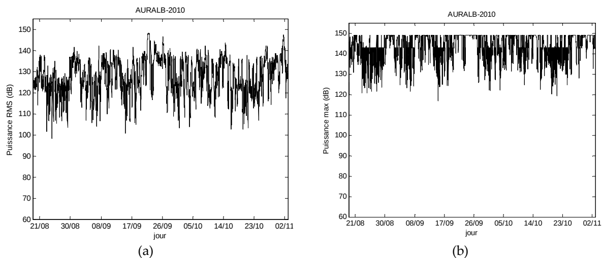
Figure 22 : évolution de la puissance au cours des enregistrements a) puissance RMS et b) puissance max
