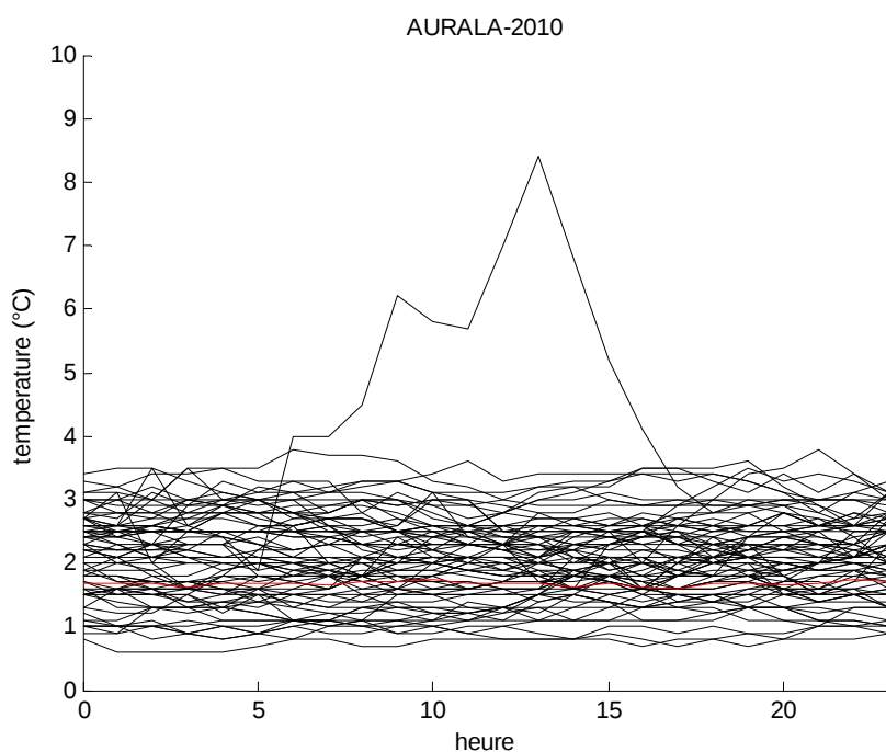
Figure 6 : évolution de la température au cours de la journée
