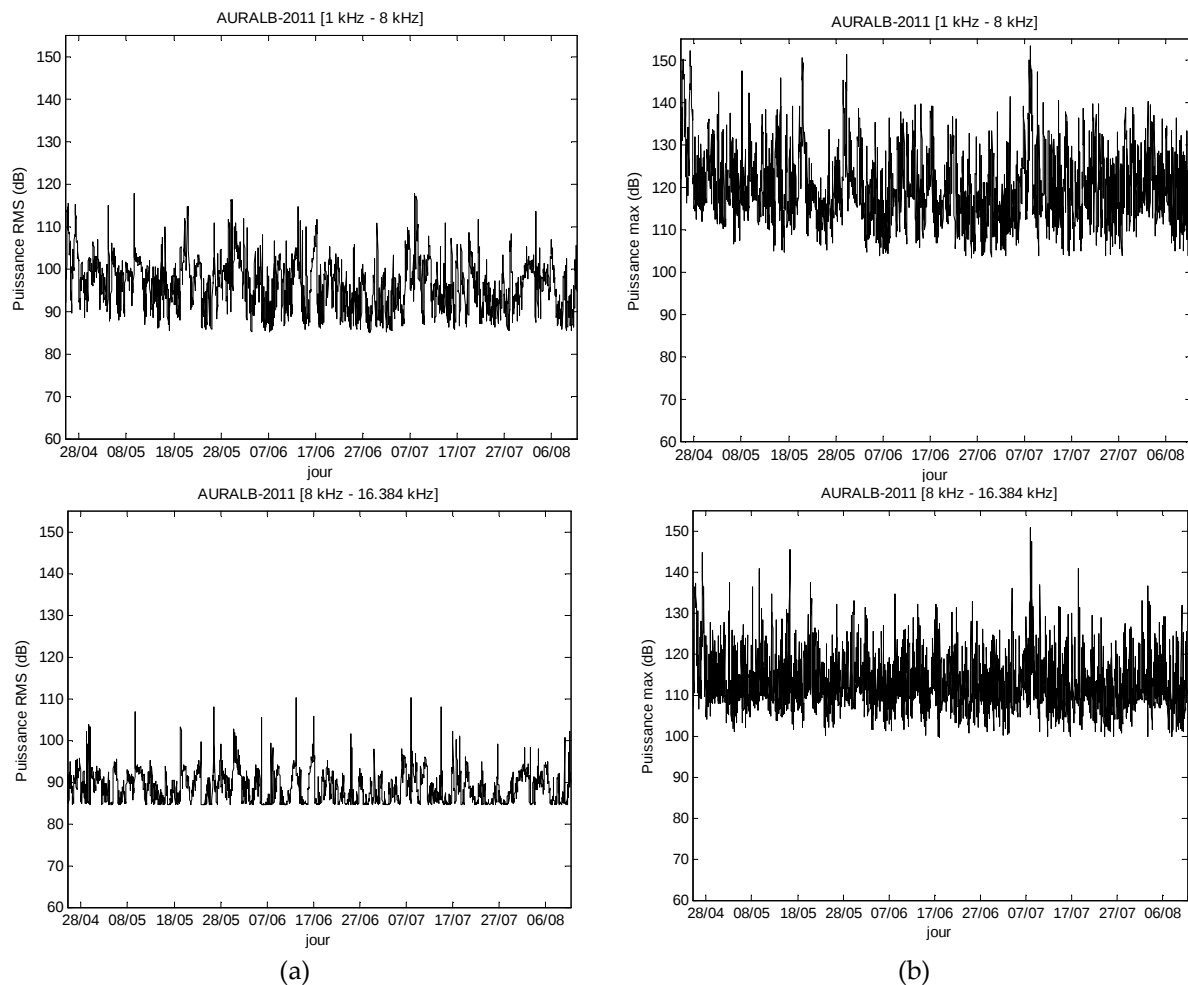
Figure 27 : évolution de la puissance au cours des enregistrements dans les différentes bandes fréquentielles a) puissance RMS et b) puissance max
