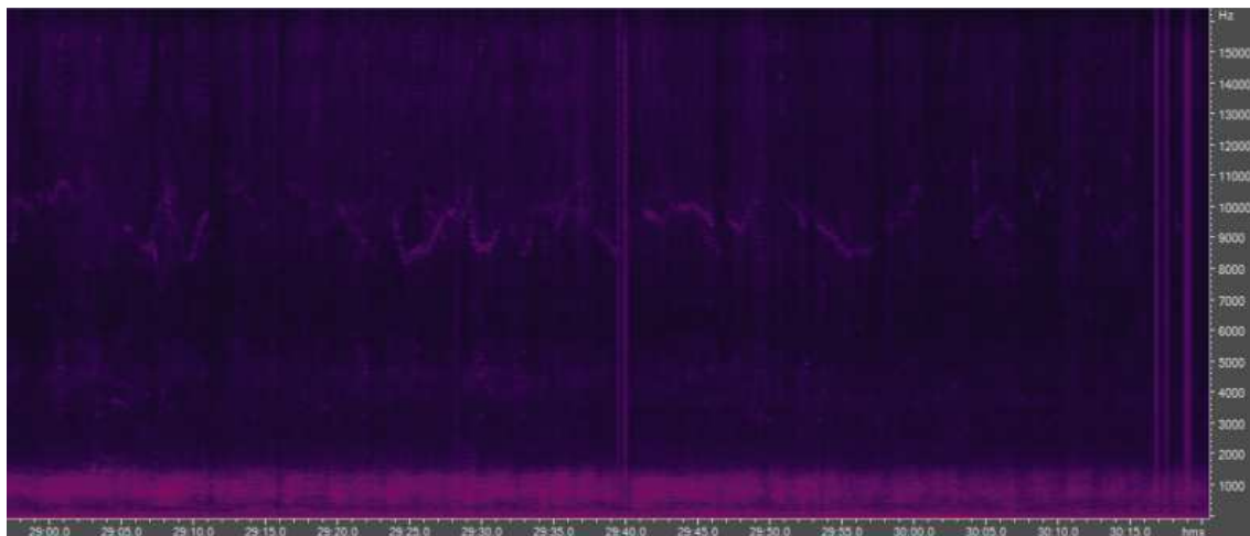
Figure 30 : clics et sifflements émis par des dauphins Extraits d'AuralA 2010, A32C0248, 30/8/2010, 01:28min40 à 01:30min21
