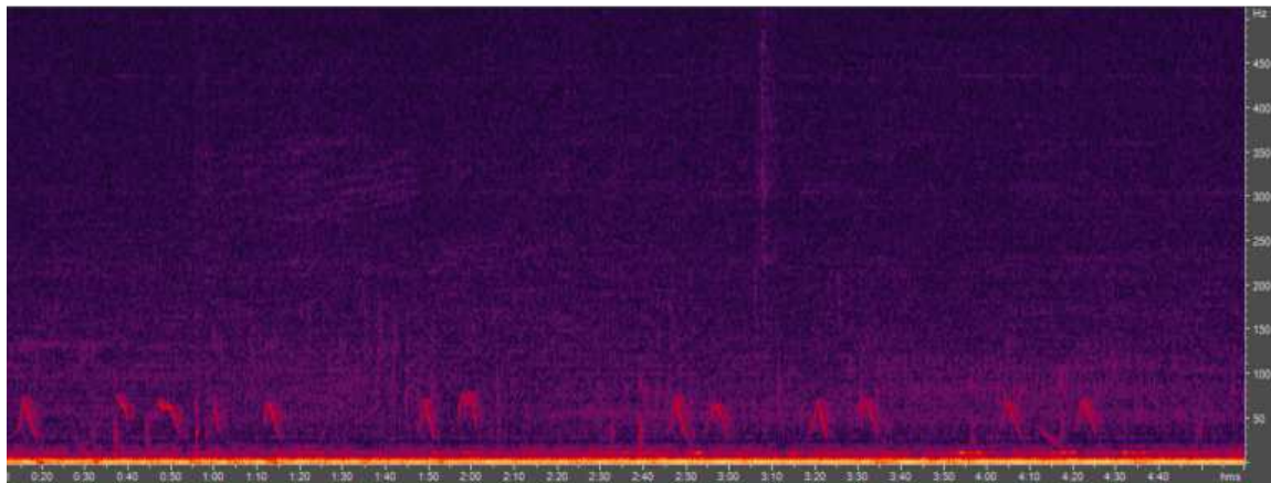
Figure 40 : vocalises de baleines bleues
