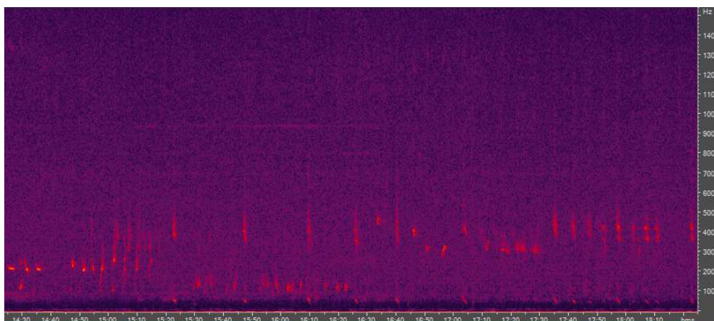
Figure 38 : vocalises de mysticètes
