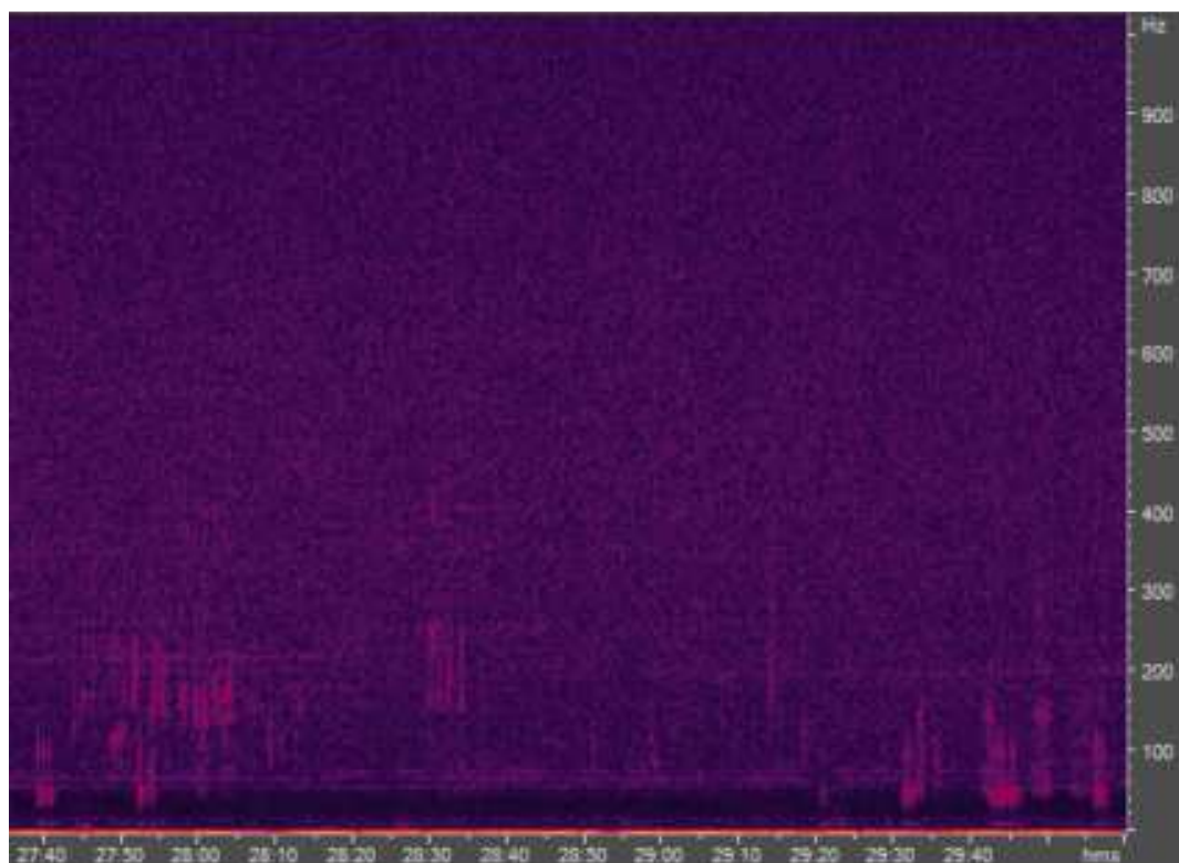
Figure 44 : vocalises de mysticète (inférieur à 300Hz)
