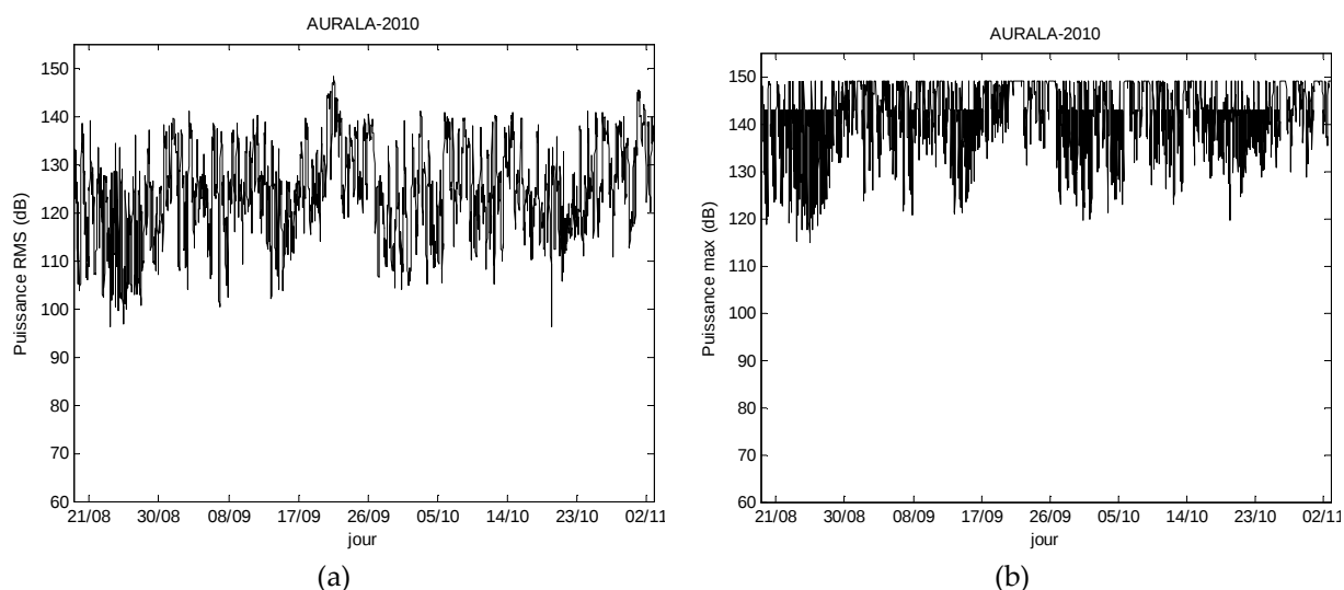
Figure 20 : évolution de la puissance au cours des enregistrements a) puissance RMS et b) puissance max
