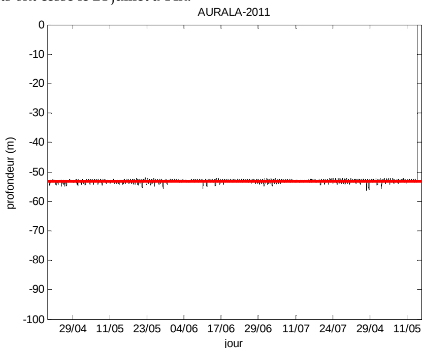
Figure 10 : profondeur pendant la période d'enregistrement
