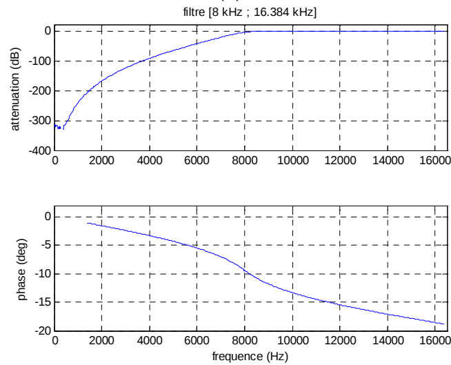
Figure 16 : réponse en fréquence et phase des filtres utilisés dans cette étude
