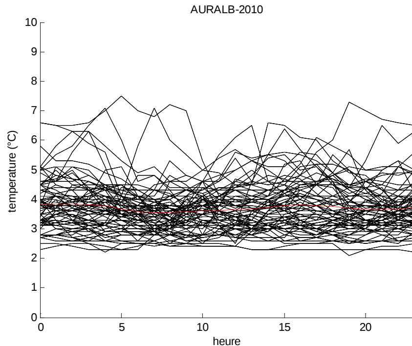
Figure 9 : Température en fonction de l'heure du jour
