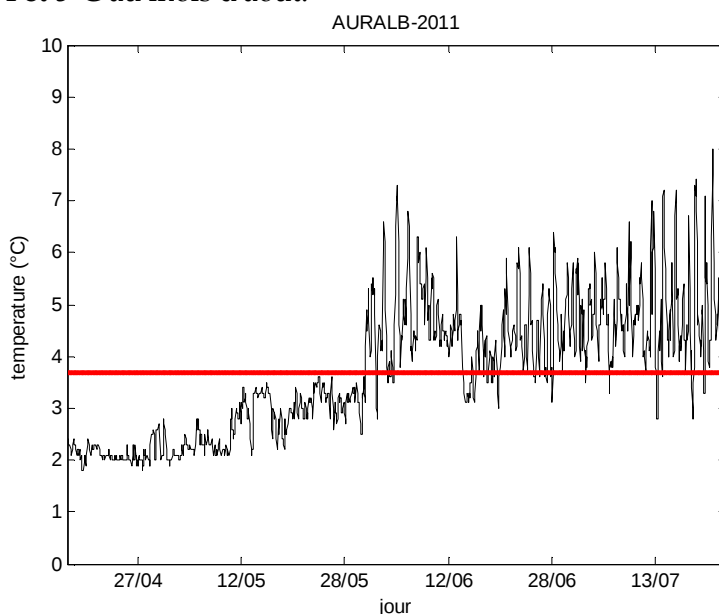
Figure 14 : température pendant la période d'enregistrement
