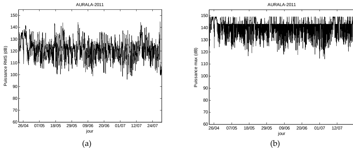
Figure 24 : évolution de la puissance au cours des enregistrements a) puissance RMS et b) puissance max
