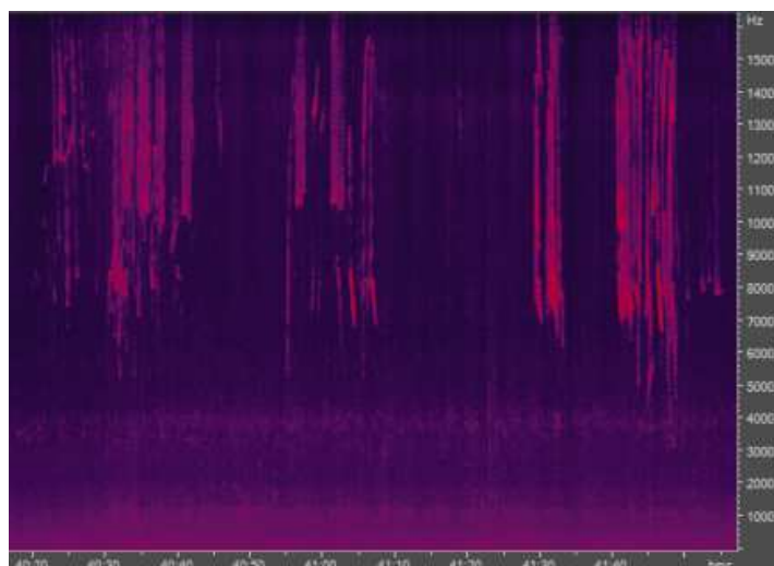
Figure 28 : sifflements de dauphins
