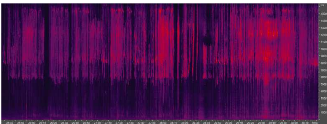
Figure 31 : plusieurs dauphins émettant des clics et des sifflements à proximité de l'hydrophone Extraits d'AuralA 2010, A32C0254, 30/8/2010, 07:27min52 à 07:30min
