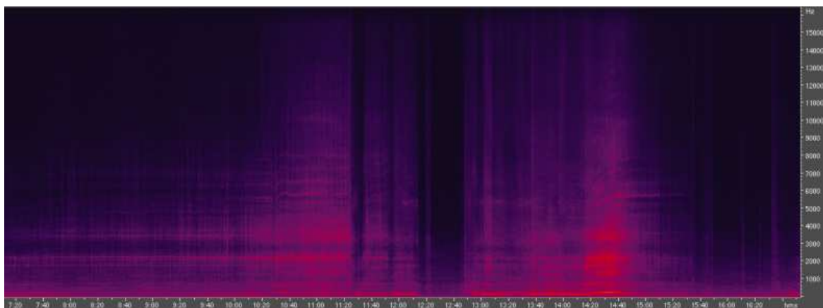
Figure 18 : bruit de bateau arrivant sur zone Extrait d'AuralA, 2011, A32C0724, 23/5/2011, 17:08min20 à 16min40
